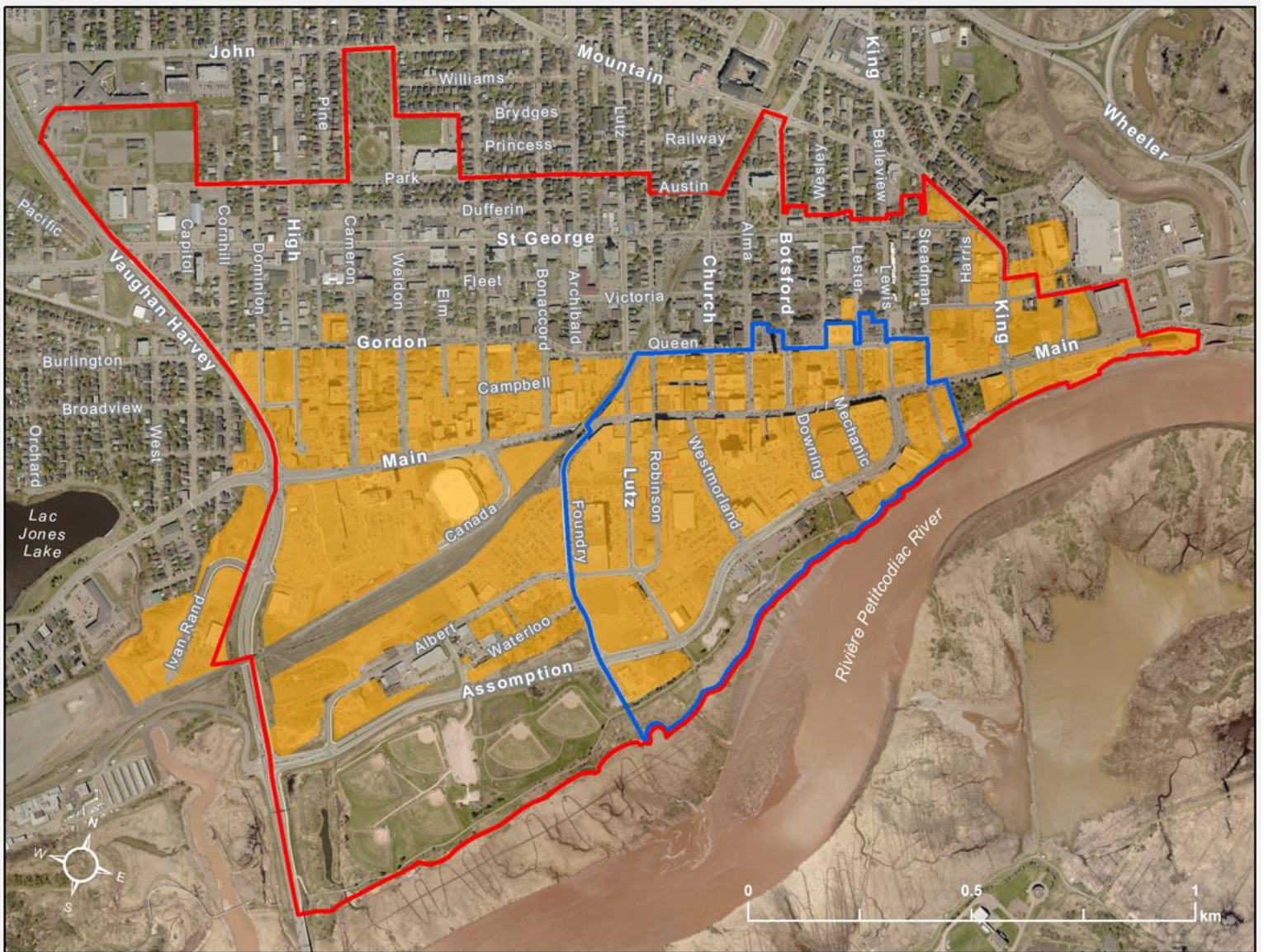
Zone d'amélioration des affaires du centre-ville Zone du quartier central des affaires Plan d'améliorations communautaires du centre-ville
